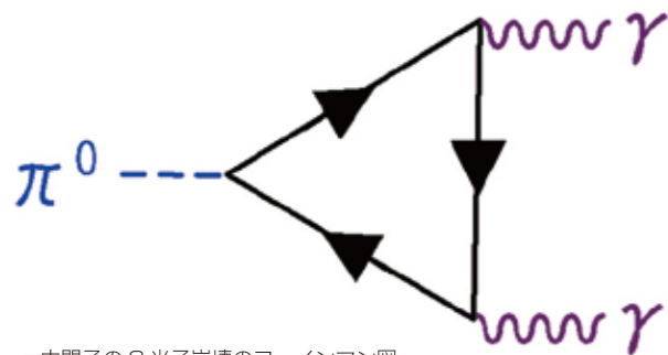
\pi 中間子の2光子崩壊のファインマン図
