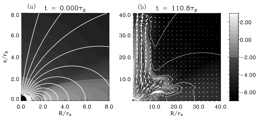
図6 非常に速く回転する（最大自転角運動量の99.995%の角運動量を持つ）ブラックホールの近傍に電流ループがある場合の GRMHD 数値シミュレーション結果（[38] より転載）．(a) t = 0 (b) t = 110.8\tau_s ．ここで、 \tau_s = r_s/c は時間の単位、 r_s はブラックホールのシュワルツシルト半径である．原点の黒い扇形はブラックホール地平面の内部、破線はエルゴ領域の表面を表す．白い実線は磁気面、矢印はプラズマの速度、濃淡はプラズマの質量密度を示している．初期の磁場は赤道面上の円 r = r_s に沿った電流ループの作る定常磁場で、赤道面上の降着円盤の初期の速度はケプラー速度（円軌道の速度）により与える．エルゴ領域と降着円盤に架かる磁気的橋はエルゴ領域において空間の引きずり効果により急速にねじられ、磁気的橋内の磁気圧が急速に高くなる．その磁気圧により磁気的橋は膨張し、ジェットを形成する．このとき、磁気的橋内の磁場は反平行になり、磁気リコネクションが起こりやすい状況となっている．現在の GRMHD シミュレーションでは抵抗はゼロとしているので、右図(b)に見られる磁気島は数値的なものである．
