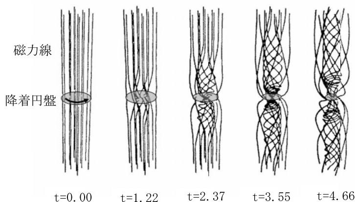
図4 柴田・内田(1986)の数値計算結果[16]。初期( t=0 )では磁場は降着円盤に垂直で一様であったが、降着円盤の回転によりねじられそのねじれが外側に伝わっている様子が見てとれる。この際、磁気圧によりプラズマは上下方向に加速され、外側向きの回転プラズマ流が形成されている。
