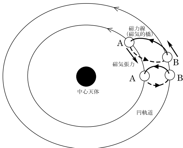
図2 磁気回転不安定性の説明。中心天体に近いほうのプラズマの塊 A は磁気的橋の磁気張力により角運動量を失い落下してゆく。逆に、外側のプラズマの塊 B は磁気張力により角運動量を得て外側にずれる。
