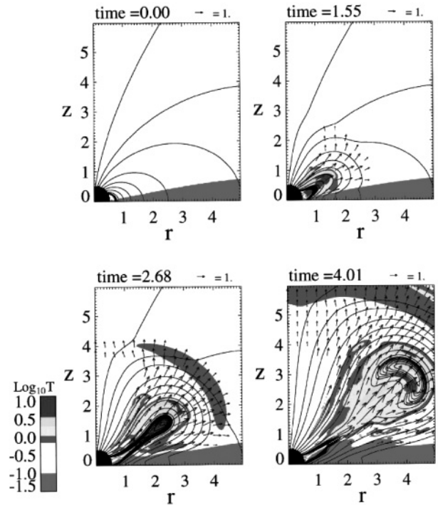
図5 林満ら (1996) の数値計算結果[18]。原点付近の黒い扇形は中心天体である星に相当する。 z=0 は赤道面に当たり、その面に沿って降着円盤は回転している。初期の回転速度はケプラー速度である。実線は磁力面、矢印は速度、濃淡は温度を示している。また、初期の磁場は原点に置いた磁気双極子で与えられる。星と降着円盤に架かる磁気的橋は降着円盤の回転によりねじられ磁気圧が大きくなる。この磁気圧により磁気的橋は膨張し、外向きのプラズマ流が生じる。また、磁気的橋が膨張すると反平行磁場が形成され、磁気リコネクションが起こりプラズマ流の追加速が起こっている。
